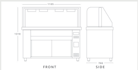
I NOKAK MFV711 (MIV711) H 1310mm W 1105mm D 700mm
