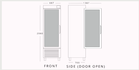
INFRICO AN501BT-CR H 2060mm W 687mm D 700mm
