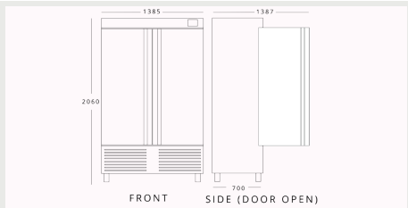
INFRICO AN1002TF H 2060mm W 1385mm D 700mm
