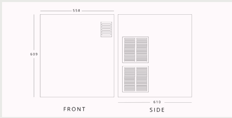
SIMAG SVD152 H 609mm W 558mm D 610mm
