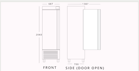
INFRICO AN501BT H 2060mm W 687mm D 700mm
