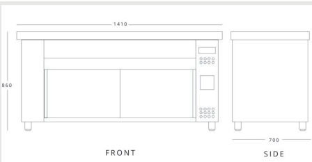
I NOKAK MDV714 (MHV714) H 860mm W 1410mm D 700mm
