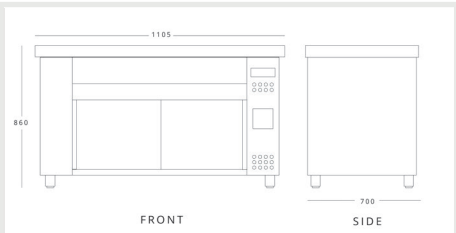
I NOKAK MDV711 (MHV711) H 860mm W 1105mm D 700mm
