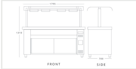
I NOKAK MRV718 (MQV718) H 1310mm W 1795mm D 700mm
