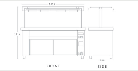
I NOKAK MRV714 (MQV714) H 1310mm W 1410mm D 700mm
