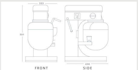
BLIZZARD FMX7 H 501mm W 333mm D 430mm
