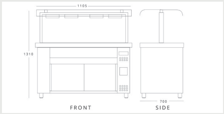
I NOKAK MRV711 (MQV711) H 1310mm W 1105mm D 700mm
