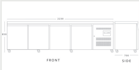
BLIZZARD LBC4NU H 850mm W 2230mm D 700mm
