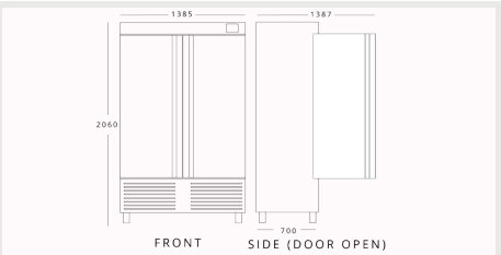
INFRICO AN1002BT H 2060mm W 1385mm D 700mm
