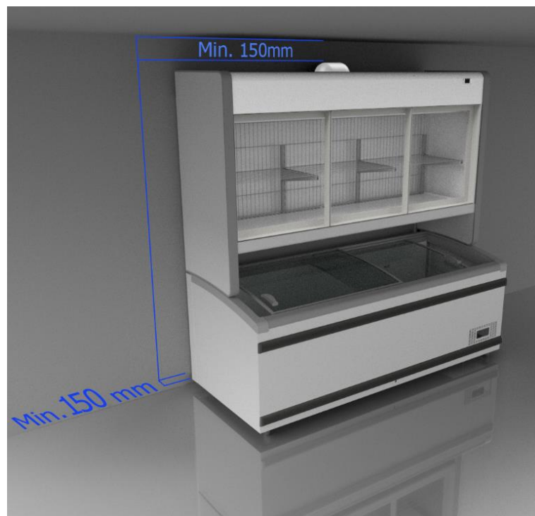
Fig.2 – Distâncias mínimas de instalação
